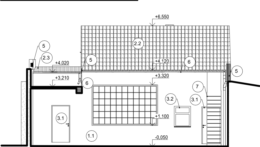
POHLED Z JIŽNÍ STRANY - ZE DVORA
