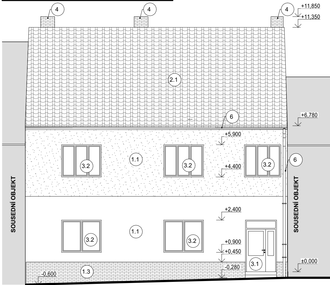
POHLED Z JIŽNÍ STRANY - Z ULICE
